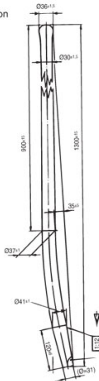
Manche DIN 20151
